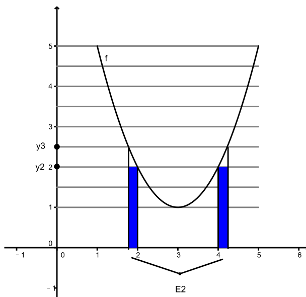
图 4: 勒贝格积分
